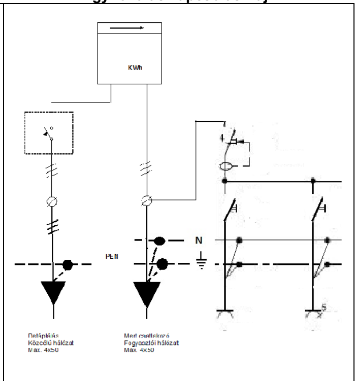
Egyvonalas kapcsolási rajz
